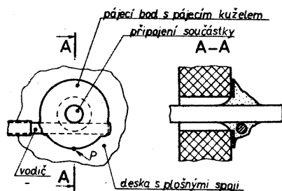
Obr. 11. Vodič rovně na osazených pájecích bodech. Vodič končí v pájecím spoji nebo se mechanicky neodděleně vede dále. V bodě P obrázku nesmí vodič přesahovat pájecí bod
